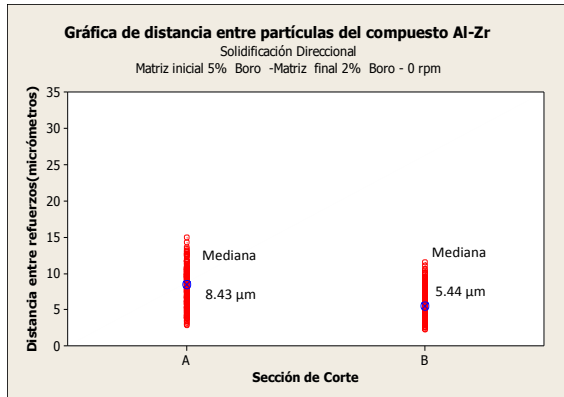
Fig. 1. Comparación por secciones de dispersión del valor de medianas ( \mu\text{m} ) para la respuesta distancia entre partículas del material AlZr con 5% de diboruro inicialmente.
